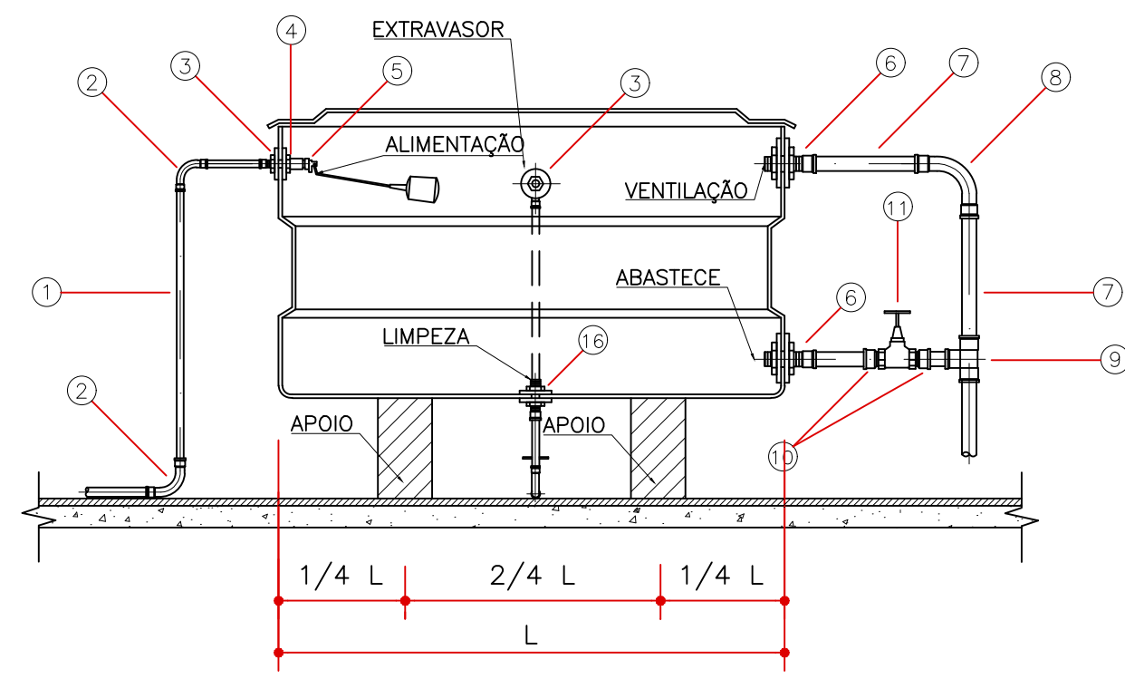
CORTE LONGITUDINAL
