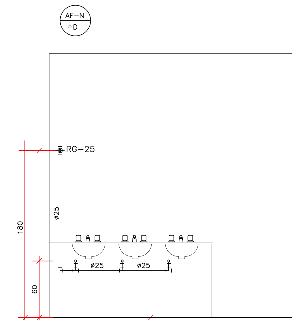
W.C. MASCULINO/FEMININO VISTA-A
