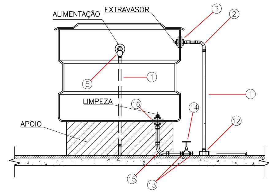
CORTE TRANSVERSAL
