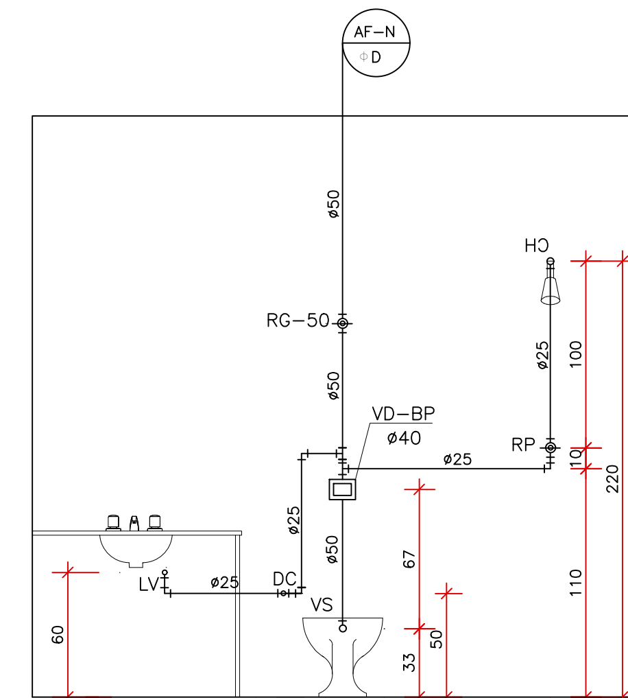
BANHO FUNCIONARIOS VISTA-A
