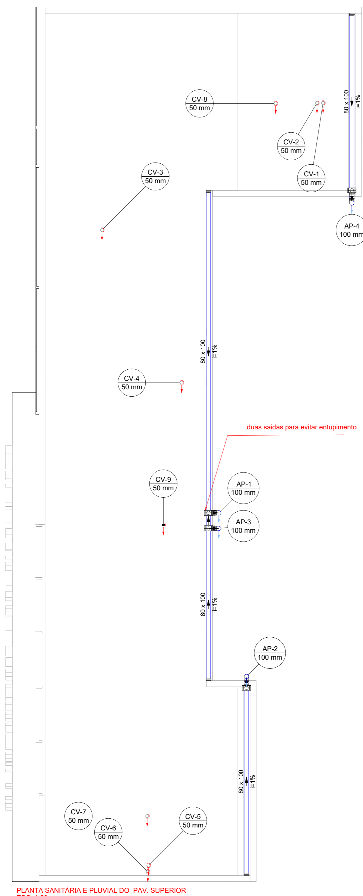
PLANTA SANITÁRIA E PLUVIAL DO PAV. SUPERIOR ESC. 1.50
