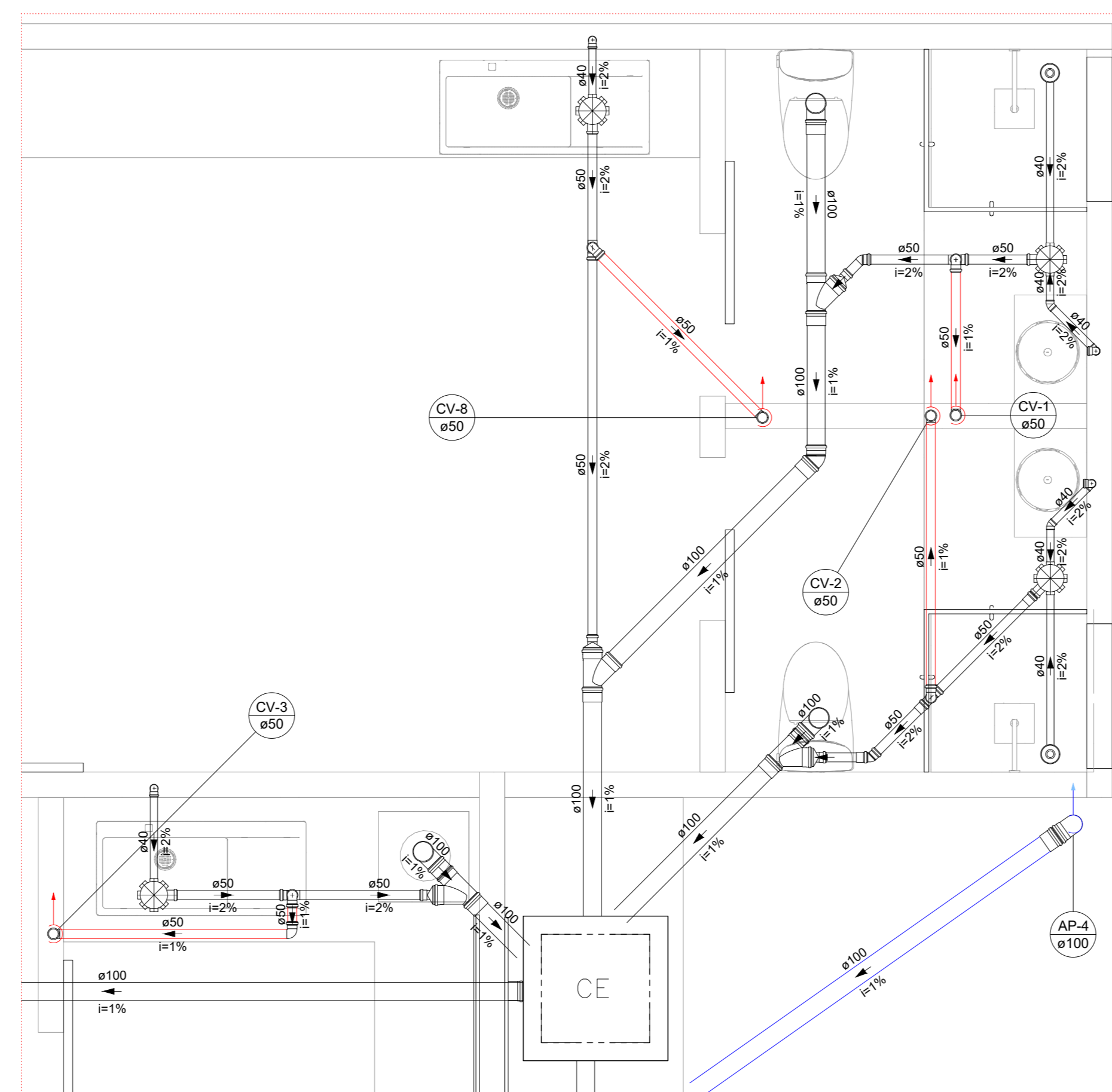
Detalhe S1 Escala 1:25
