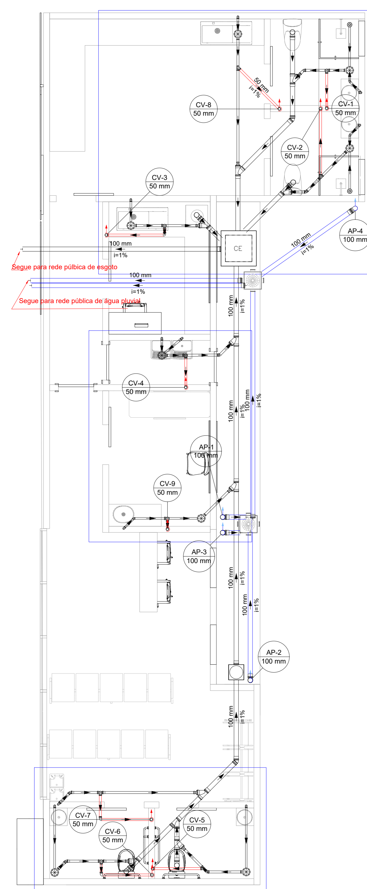
PLANTA SANITÁRIA E PLUVIAL DO TERREO ESC. 1.50
